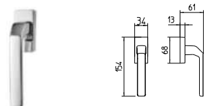
1602/DK MARTELLINA DK drehkipp system
