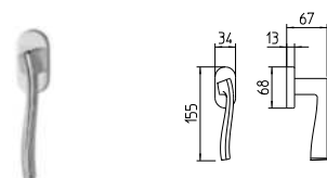
1482/DK MARTELLINA DK drehkip system
