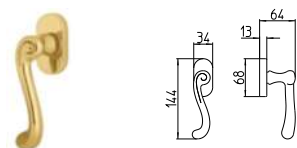
442/DK MARTELLINA DK drehkip system
