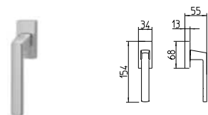
1292/DK MARTELLINA DK drehkipp system
