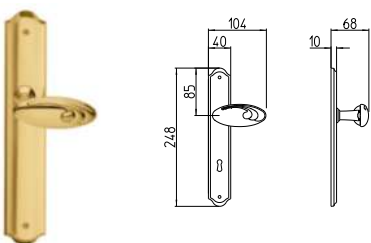
1110 MANIGLIA PER PORTA CON PIASTRA door-handle on back plate
