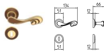
1121 MANIGLIA PER PORTA CON ROSETTA door-handle on rose
