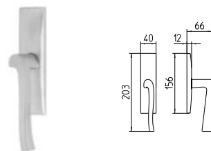
1072/M CREMONESE IMPUGNATURA MANIGLIA window lever-handle
