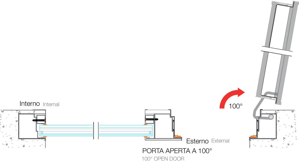
SEZIONE ORIZZONTALE HORIZONTAL SECTION
