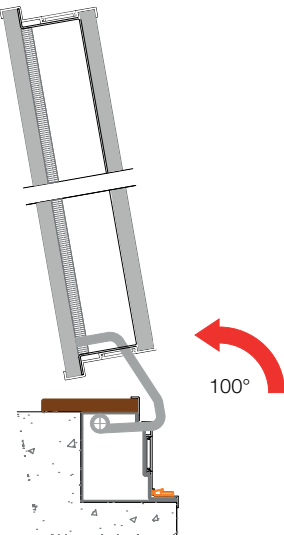
SEZIONE ORIZZONTALE HORIZONTAL SECTION
