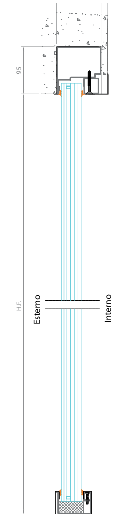
SEZIONE VERTICALE FIANCOLUCE VERTICAL SIDE PANEL SECTION
